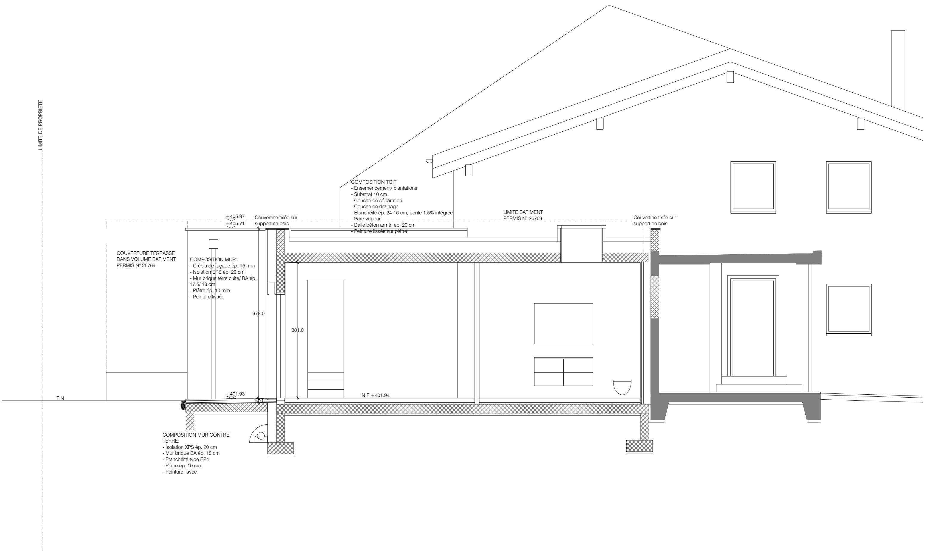
Coupe AA
